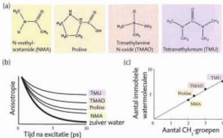
Figuur 4 (a) Structuurformules van de amfifiele moleculen die in het experiment gebruikt zijn. (b) We hebben het anisotropieverval van watermoleculen bepaald in een viertal oplossingen van dezelfde concentratie (5 mol per liter). In zuiver water is de reoriëntatietijd van watermoleculen 2,5 ps zoals op te maken is uit het feit dat de anisotropie met deze tijdsconstante vervalft. In de vier oplossingen komen twee soorten watermoleculen voor: snel draaiende moleculen en langzaam draaiende moleculen. De langzaam roterende moleculen zorgen ervoor dat de anisotropie slechts gedeeltelijk vervalft tot een plateau. De hoogte van het plateau geeft het percentage immobile watermoleculen. (c) Aantal immobile watermoleculen per amfifiel molecuul uitgezet tegen het aantal methylgroepen in het molecuul. Proline bevat geen methylgroepen. Om het molecuul toch een plaats te geven in de grafiek hebben we gekeken naar het aantal CH-groepen. Dit zijn er 7, wat overeenkomt met 2,3 methylgroepen.
