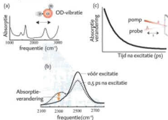
Figuur 2 (a) Het infraroodspectrum van HDO vertoont een resonantie bij 2500 cm -1 als gevolg van de vibratie van de OD-groep van het molecuul. (b) Aangeslagen HDO-moleculen kunnen we waarnemen in het spectrum doordat deze moleculen een lagere resonantiefrequentie hebben dan moleculen in de niet-aangeslagen toestand. (c) Door de absorptieverandering bij 2300 cm -1 te meten als functie van de tijd tussen twee pulsen kunnen we de levensduur van de OD-vibratie bepalen.
